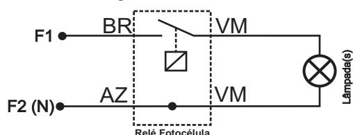
Esquema Elétrico 1
