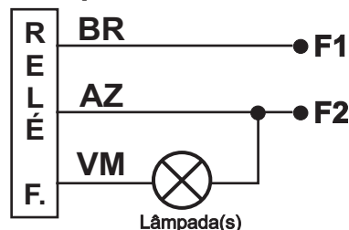
Esquema Elétrico 2
